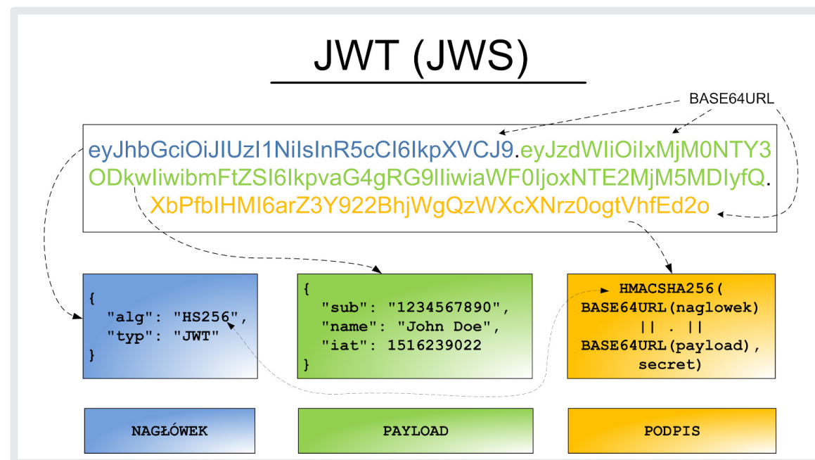
Rysunek 1. Przykład podstawowego JWT
