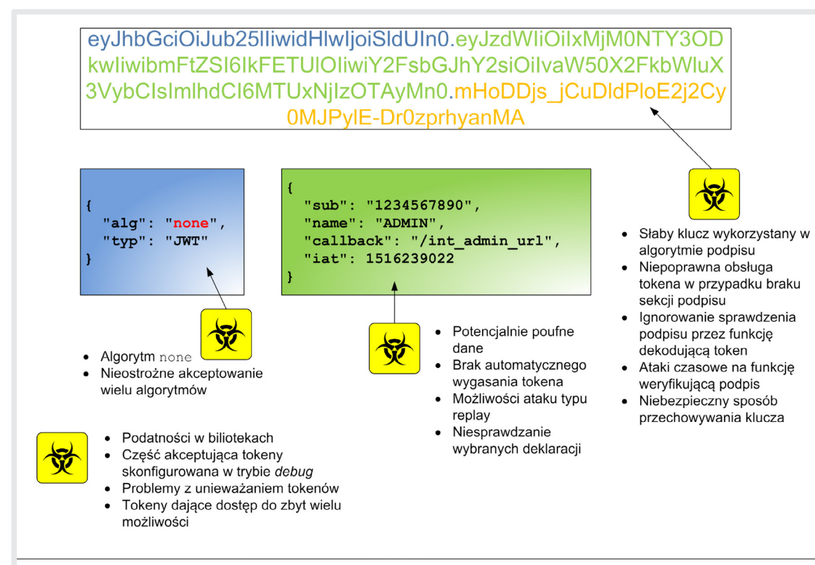
Rysunek 4. Zestawienie problemów bezpieczeństwa w JWT (JWS)
