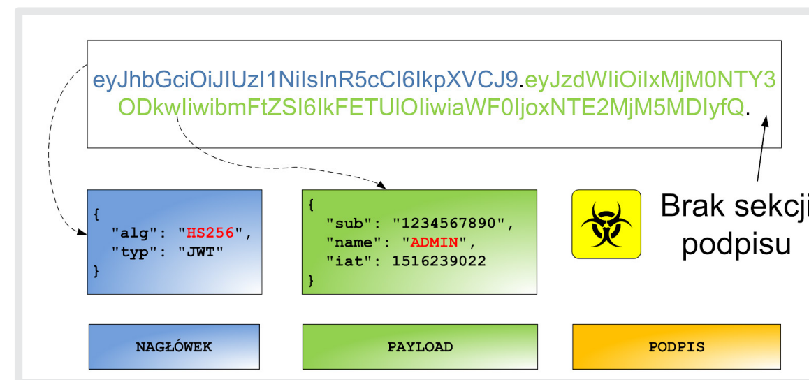
Rysunek 3. Brak sekcji podpisu, mimo wskazania algorytmu w nagłówku
