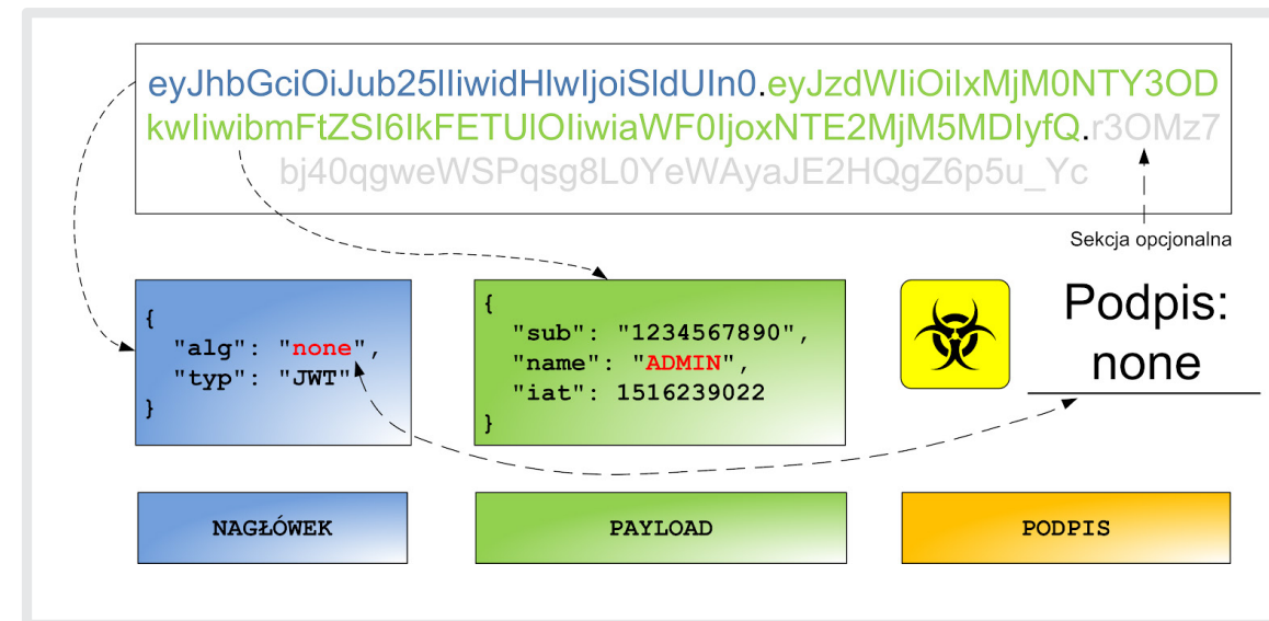
Rysunek 2. Algorytm none
